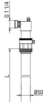
Fig. 12: Type SDL-2 DN15
